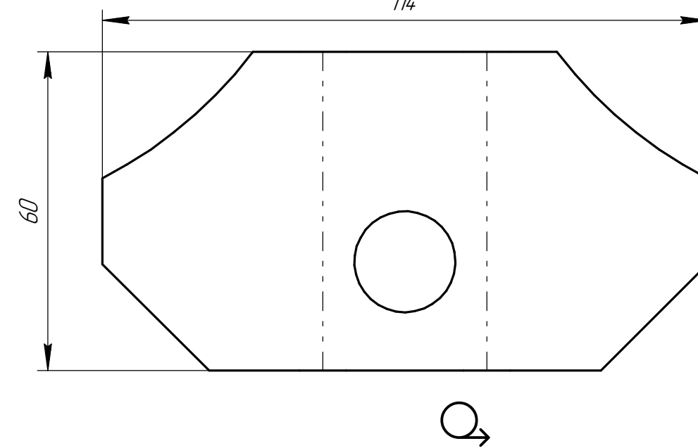
Дет. поз. 3 (1:1)
