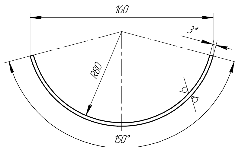
Дет. поз. 5 (1:2,5)
