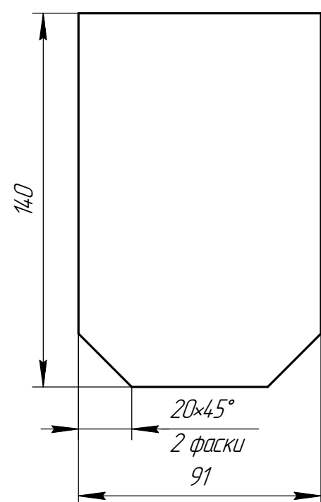
Дет. поз. 2
