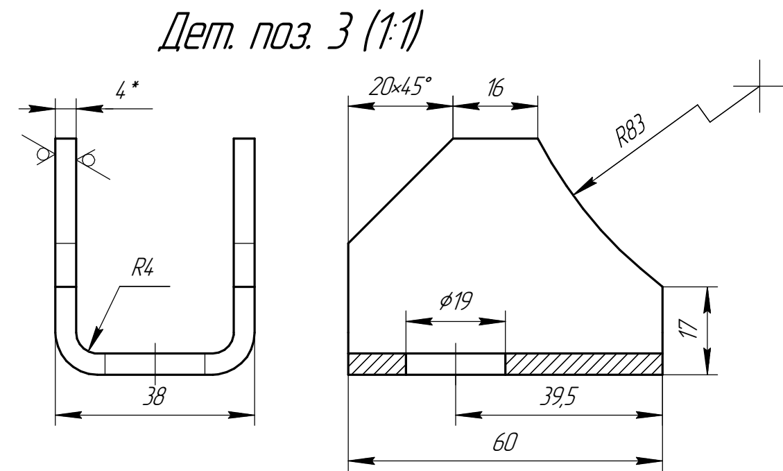
Дет. поз. 3 (1:1)
